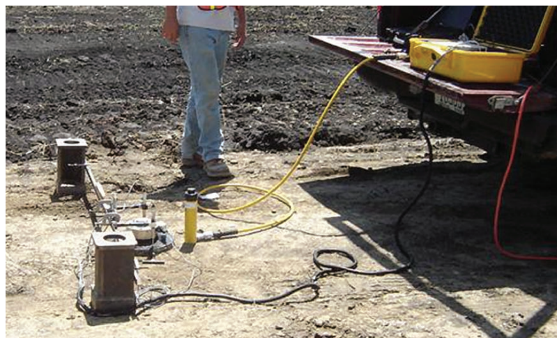
Подготовка к штамповым испытаниям
