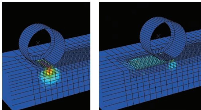
Высокая амплитуда передается глубже в грунт
