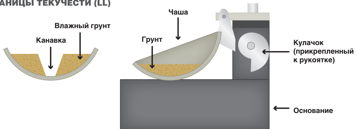
Простое испытательное устройство для определения границы текучести
