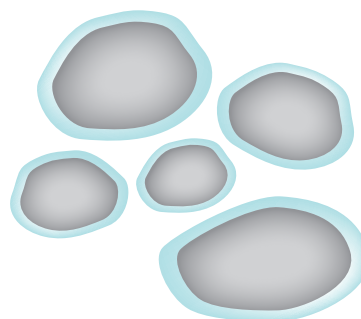
Гигроскопическая вода
